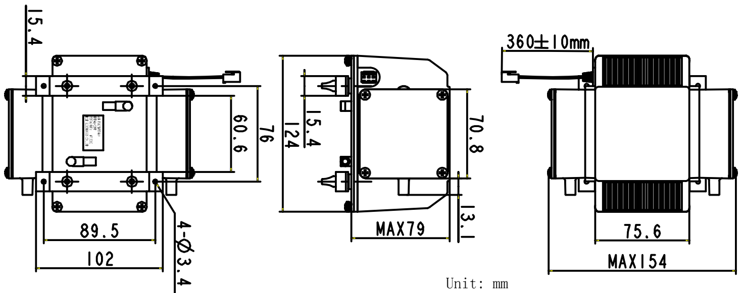
產品尺寸: Dimension
